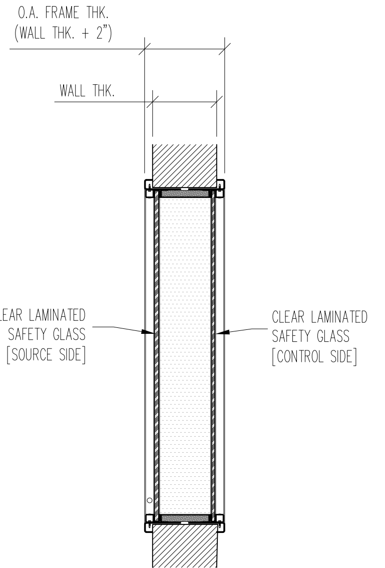
SECTION A-A
